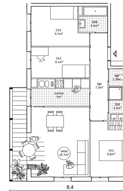
Logement 4P
