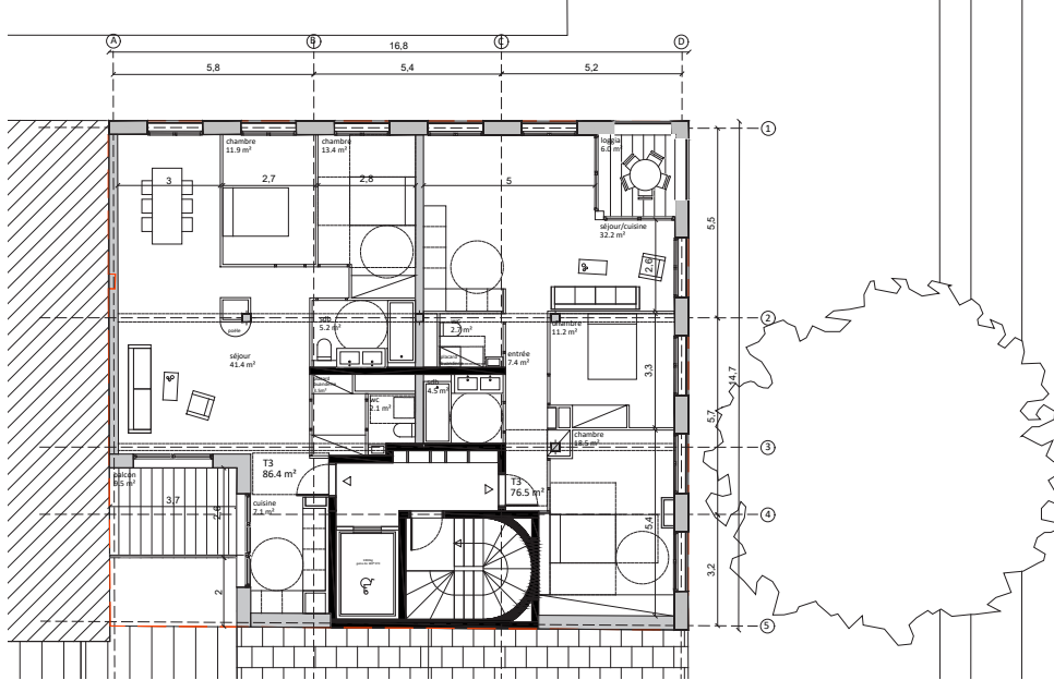
étage logements
