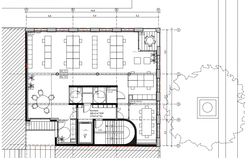
plateau bureaux
